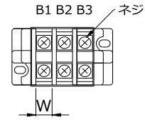
ブレーキ端子台
