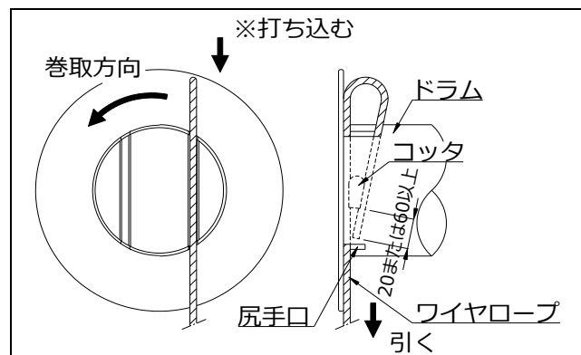
ワイヤロープの取付け（横尻手）
