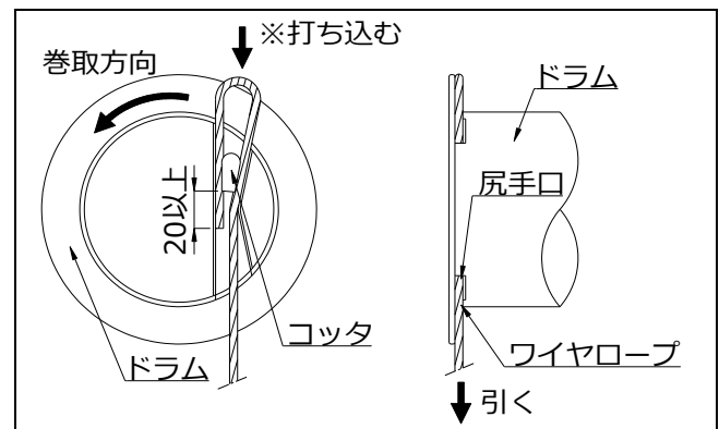
ワイヤロープの取付け（MA-3, MA-5）
