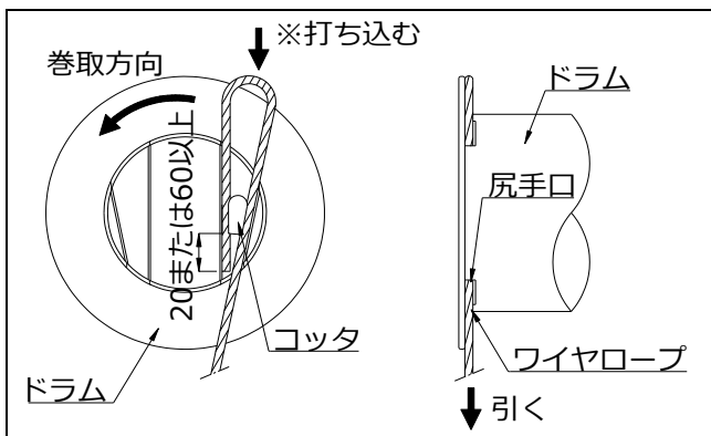
ワイヤロープの取付け（縦尻手）
