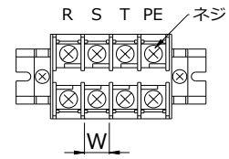
電源端子台
